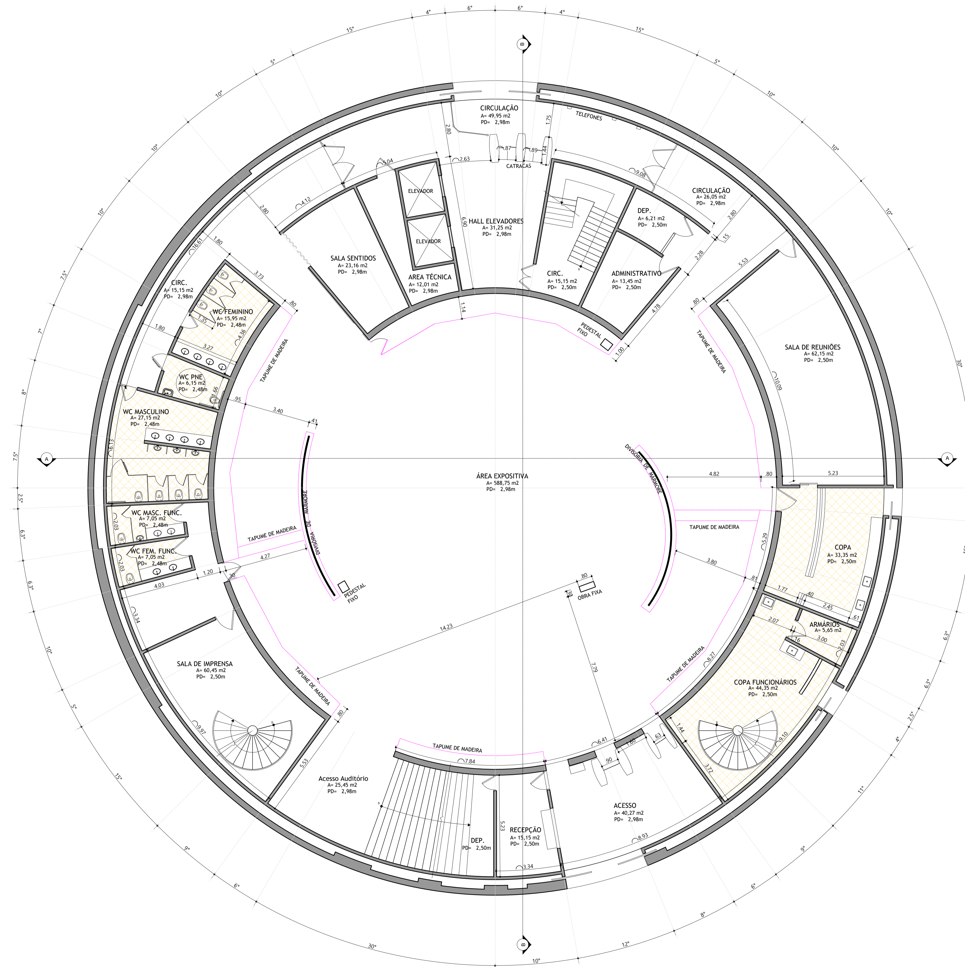
PLANTA DE SITUAÇÃO ATUAL ESC.: 1:100
