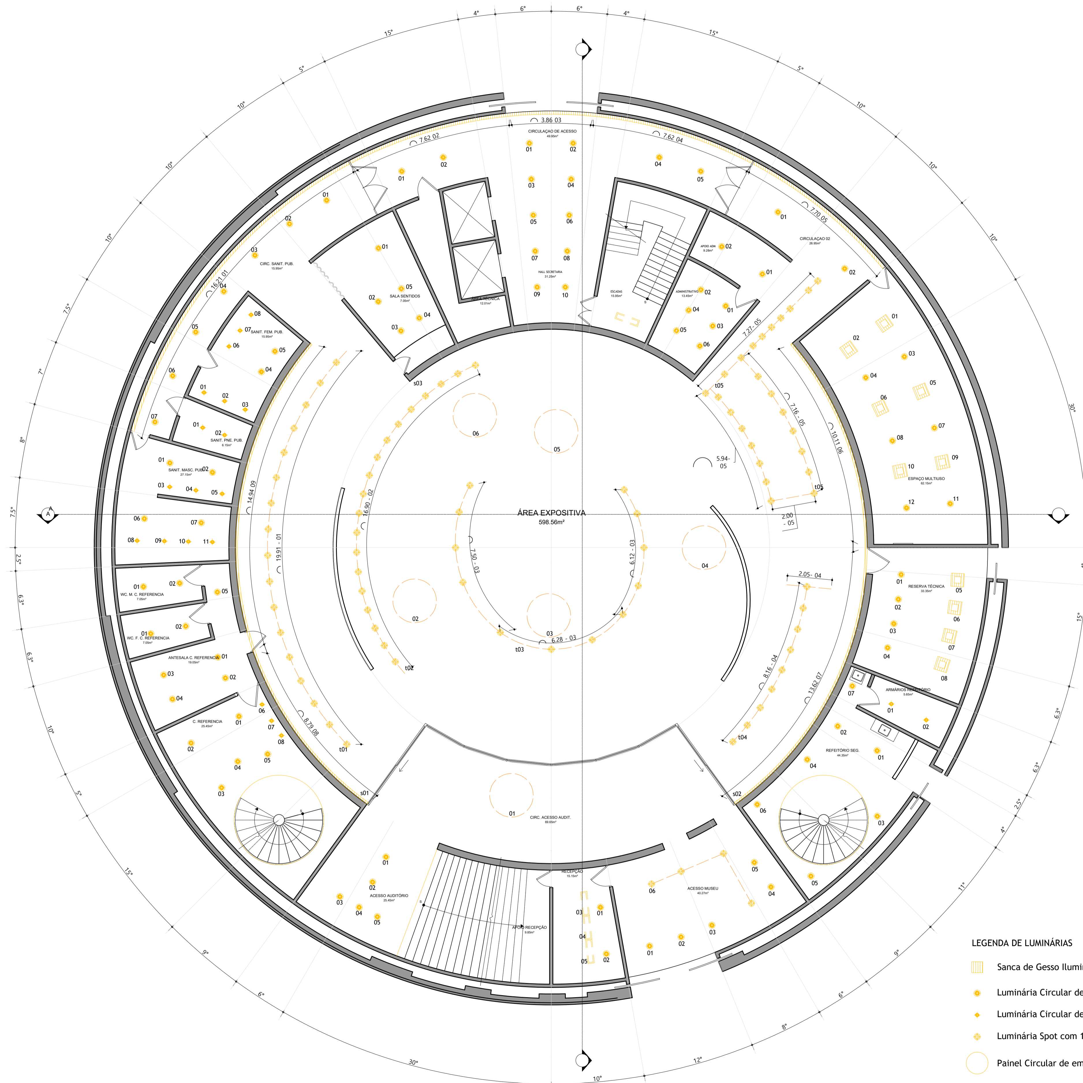
PLANTA DE LUMINOTÉCNICA ATUAL ESC.: 1:100
