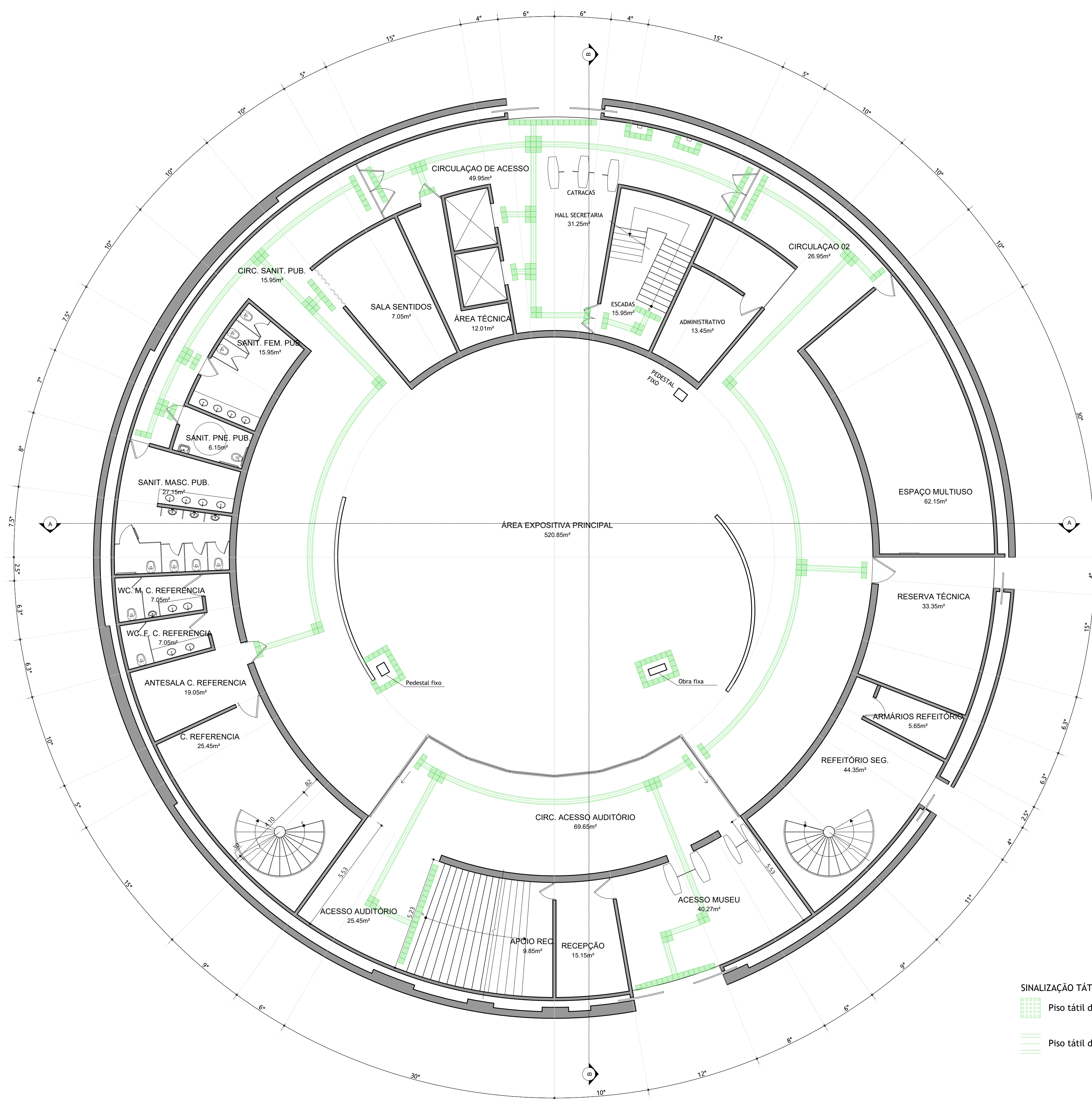
PLANTA DE ACESSIBILIDADE ESC.: 1:100
