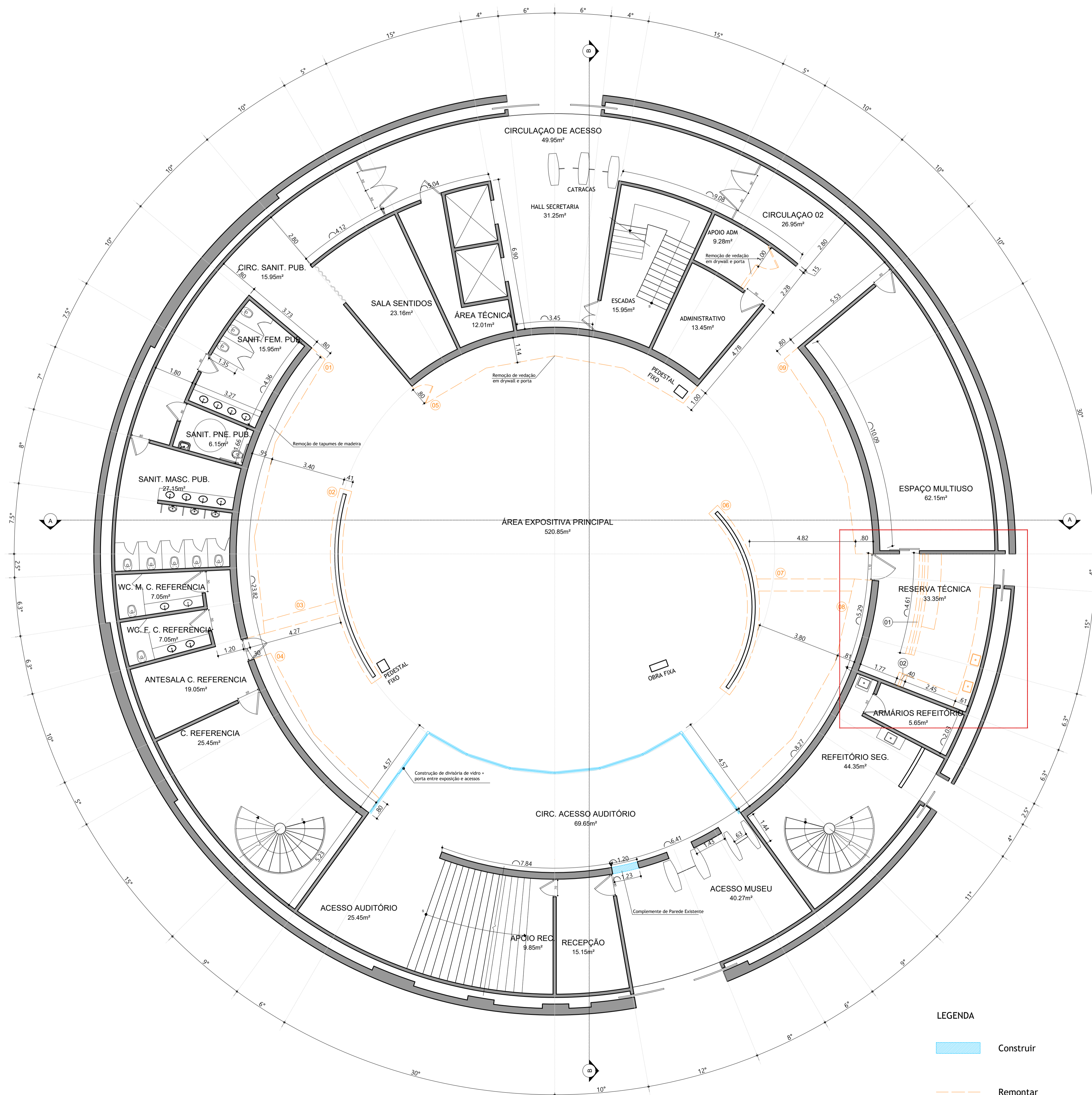
PLANTA DE REFORMA-DEMOLIR E CONSTRUIR ESC.: 1:100
