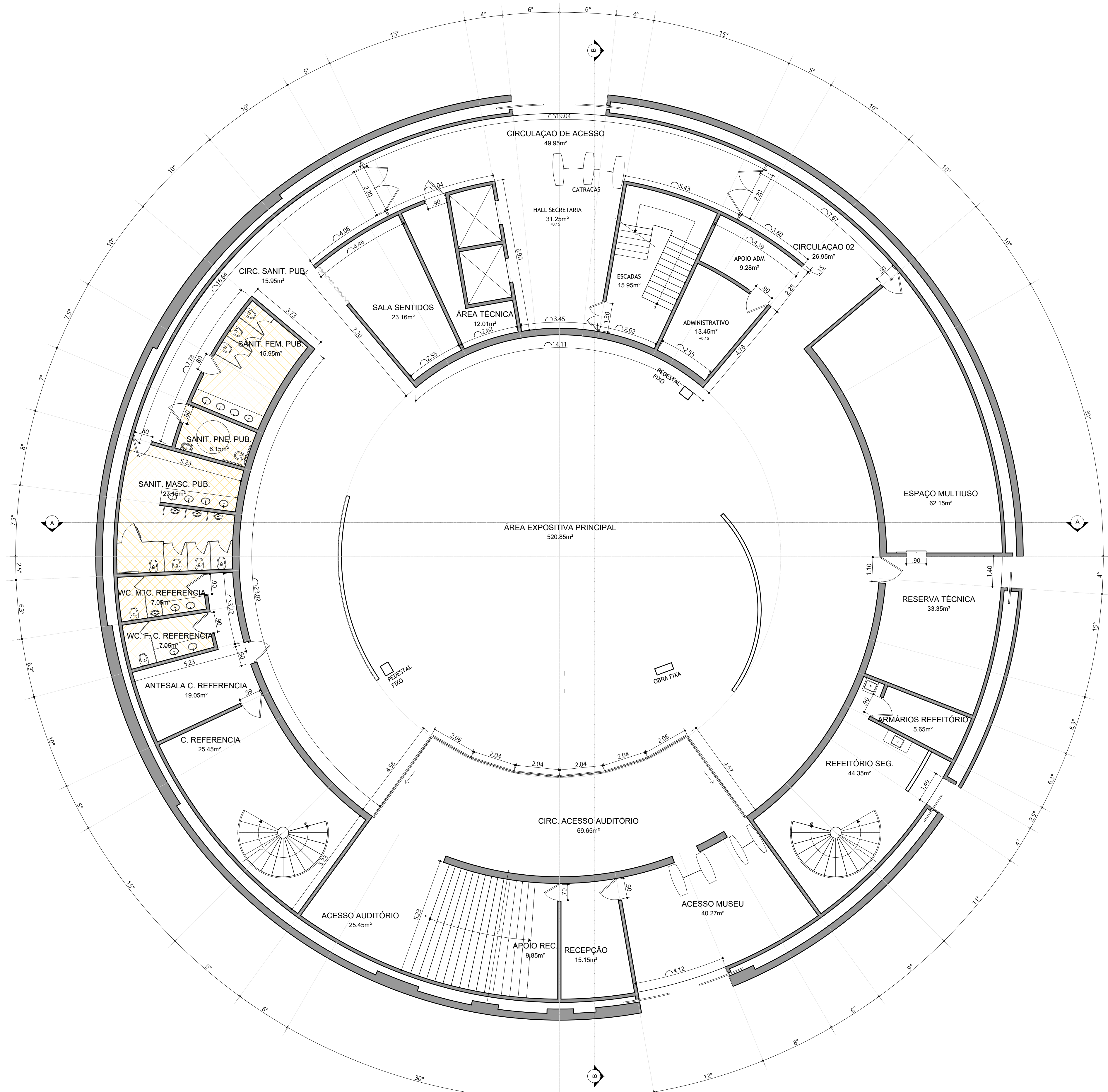
PLANTA DE LAYOUT PROPOSTO ESC.: 1:100
