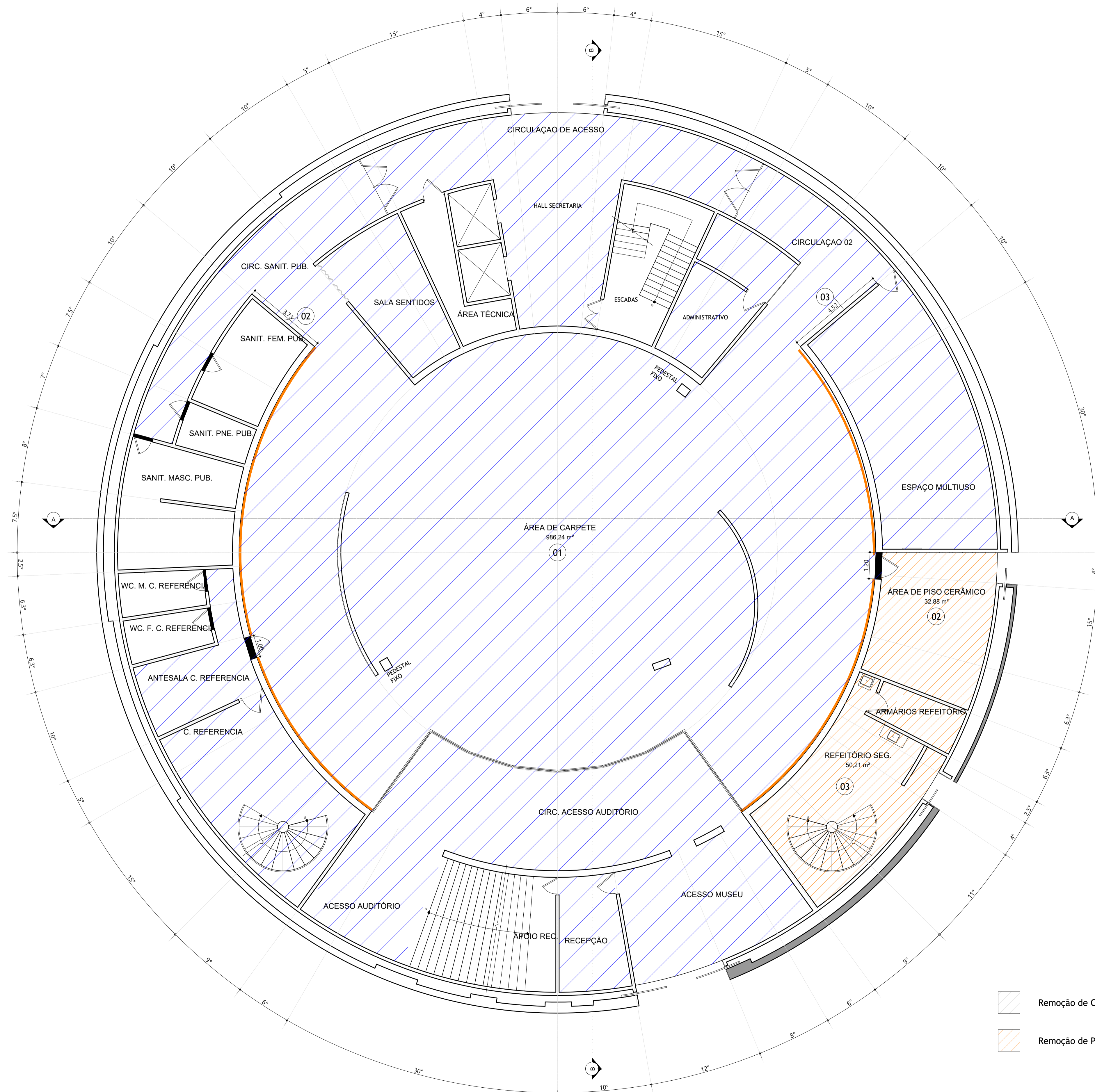
PLANTA DE REMOÇÃO DE PISO - MEMÓRIA DE CÁLCULO ESC.: 1:100
