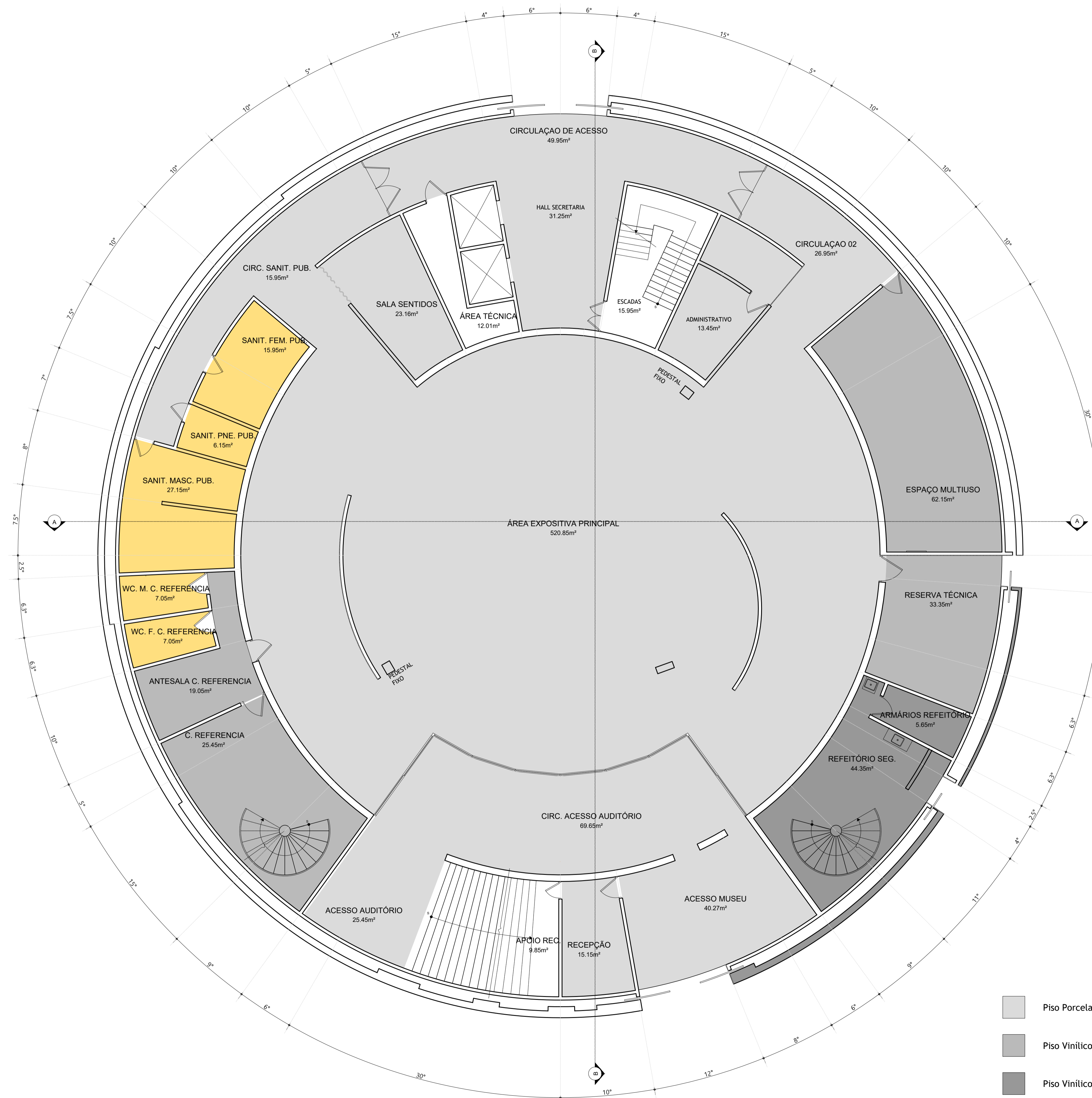
PLANTA DE REFORMA-PISO ESC.: 1:100
