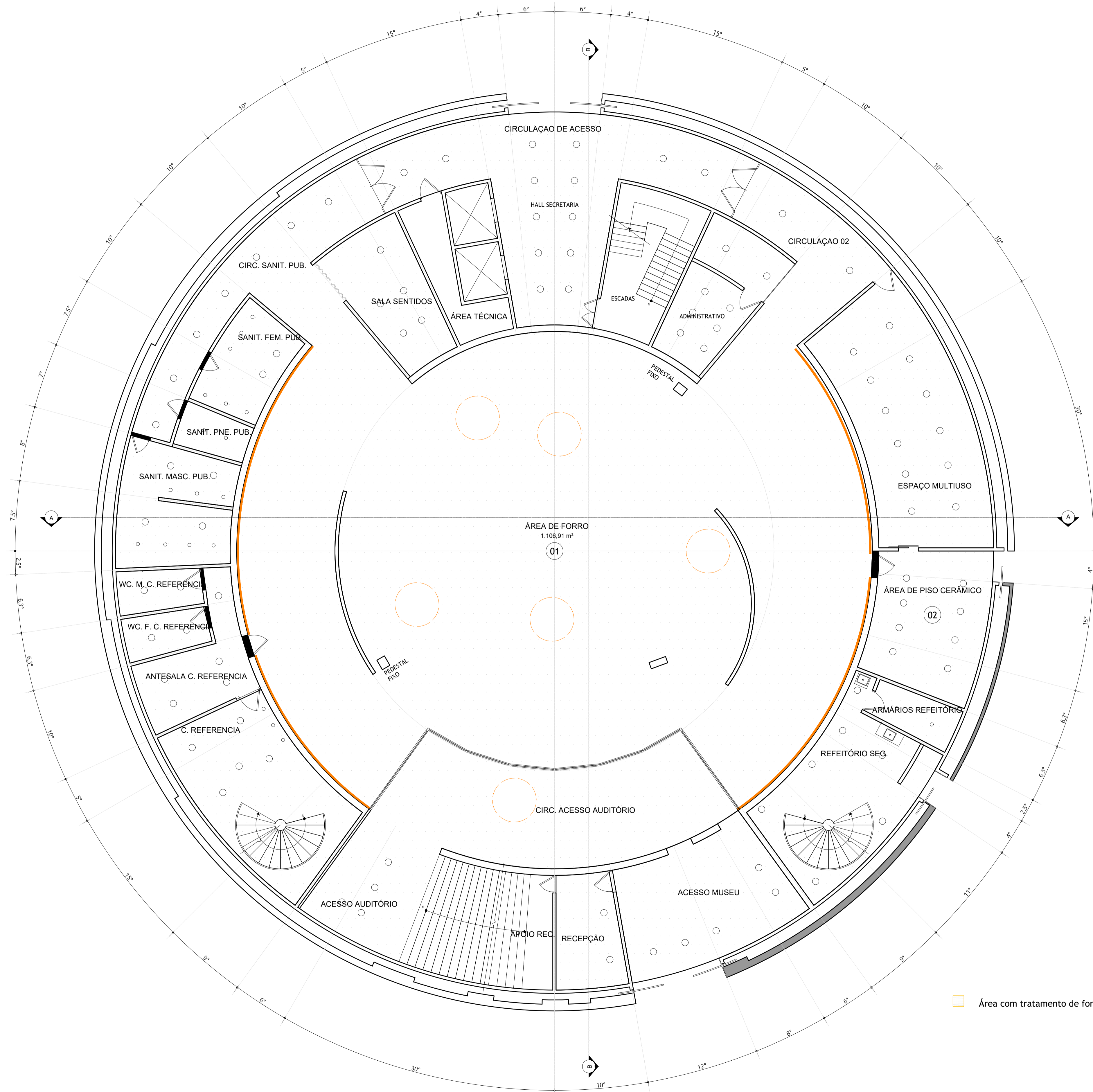
PLANTA DE FORRO - MEMÓRIA DE CÁLCULO ESC.: 1:100
